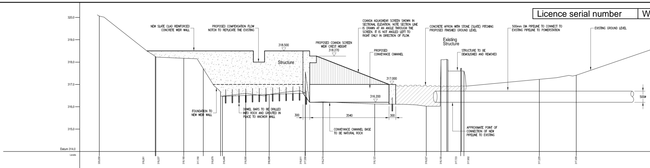
Section A-A
