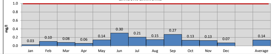
Effluent ammonia
