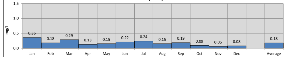
Effluent AOX
