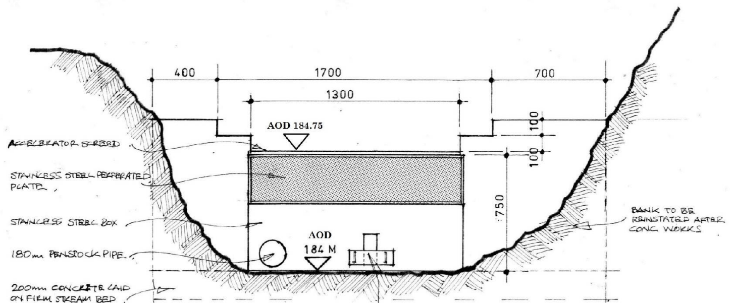
Y-Y 1:20
