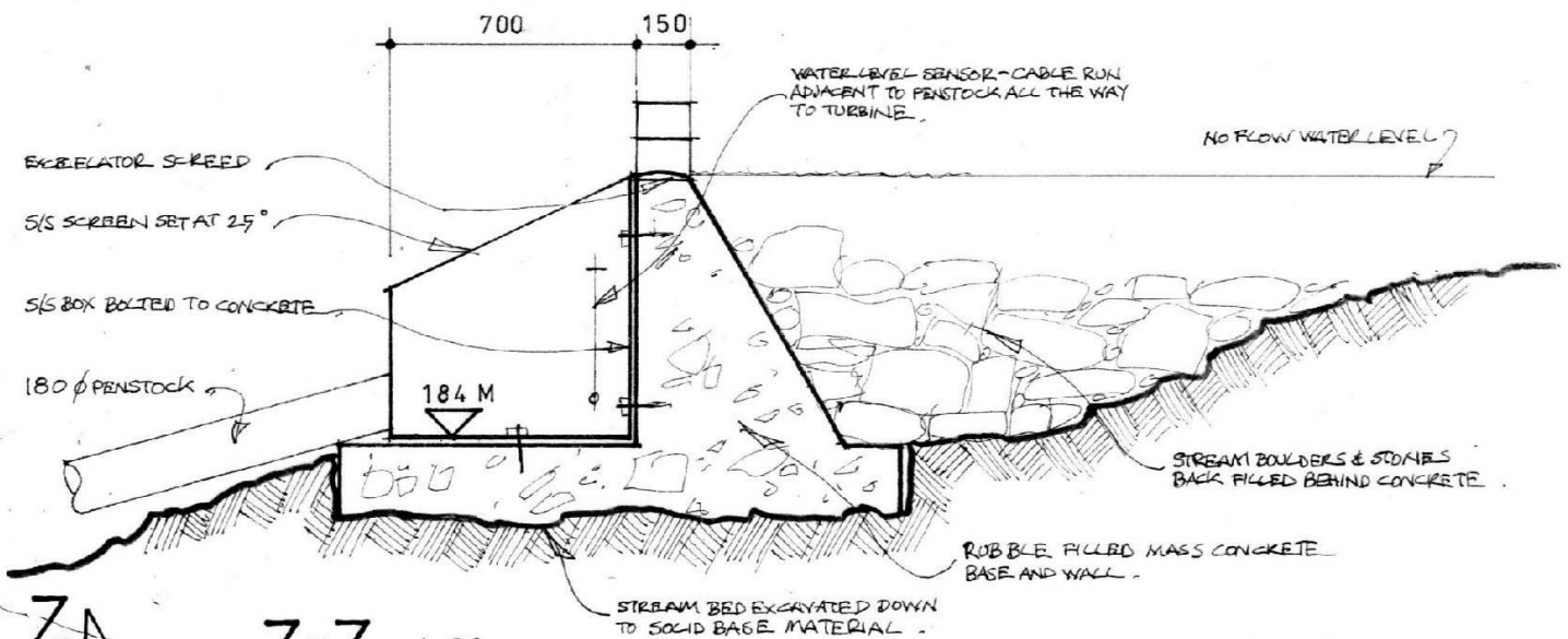
Z-Z 1:20
