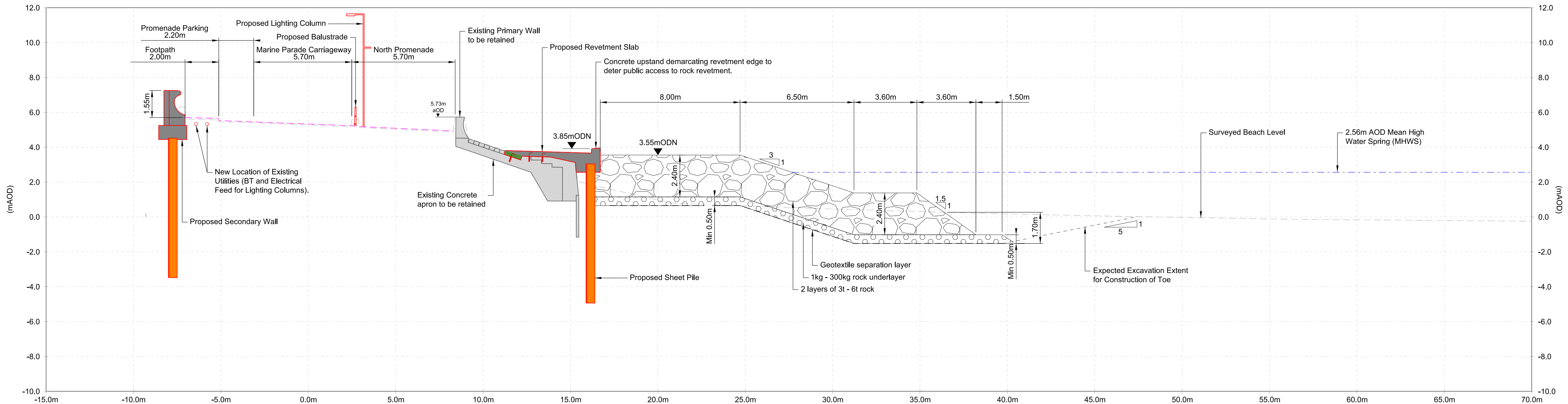
Section D-D
