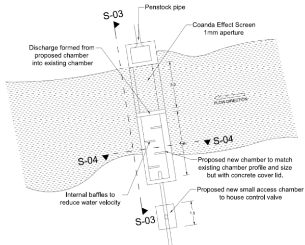
01 SITE LAYOUT 1:100
